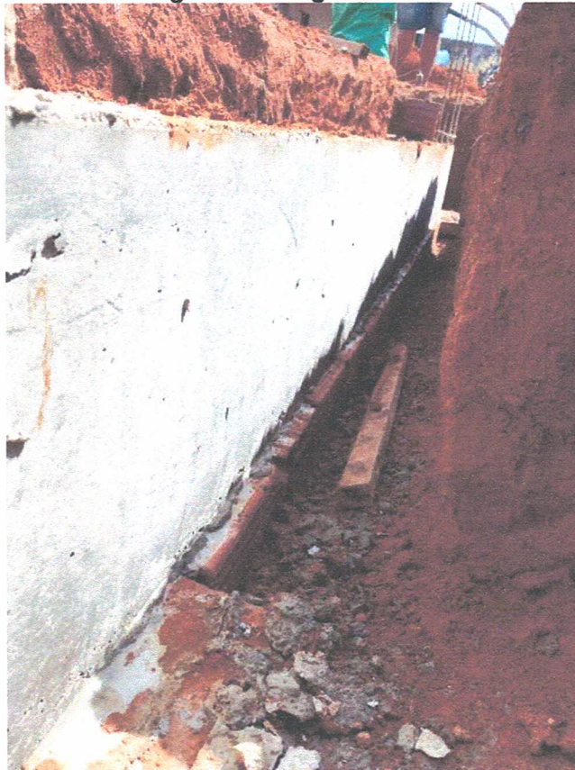
Imagem 10 – Impermeabilização da viga baldrame
