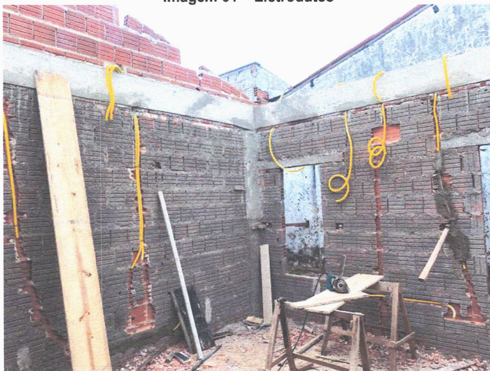
Imagem 01 – Eletrodutos
